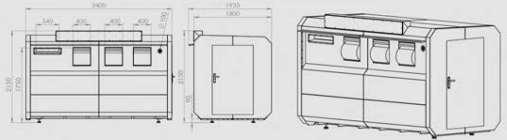
3.SINIF ATIK GETİRME MERKEZİ TEKNİK ÖLÇÜLERİ
