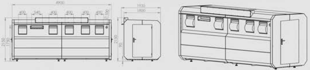
2.SINIF ATIK GETİRME MERKEZİ TEKNİK ÖLÇÜLERİ
